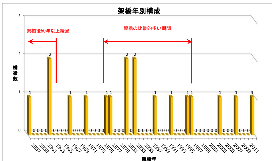
図. 3-3 架橋年別構成
