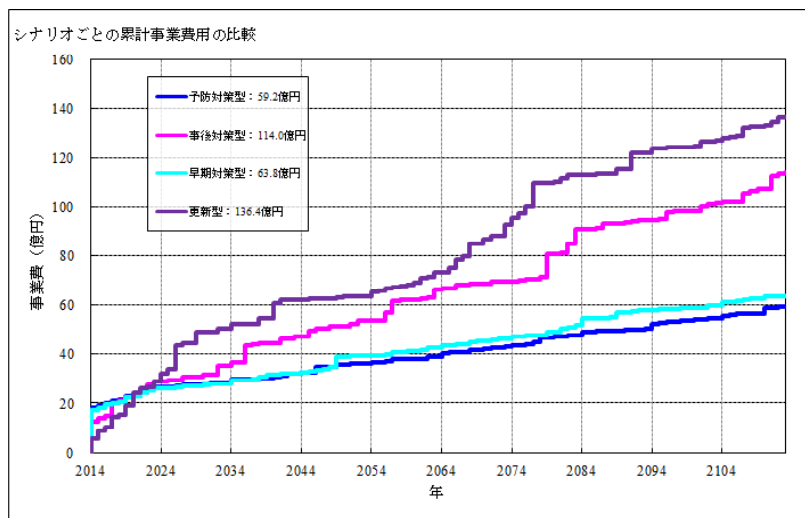
図. 11-2 シナリオごとの累計事業費
