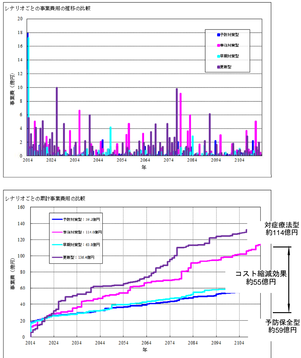
図. 14-1 対症療法型と予防保全型との累計事業費の比較
