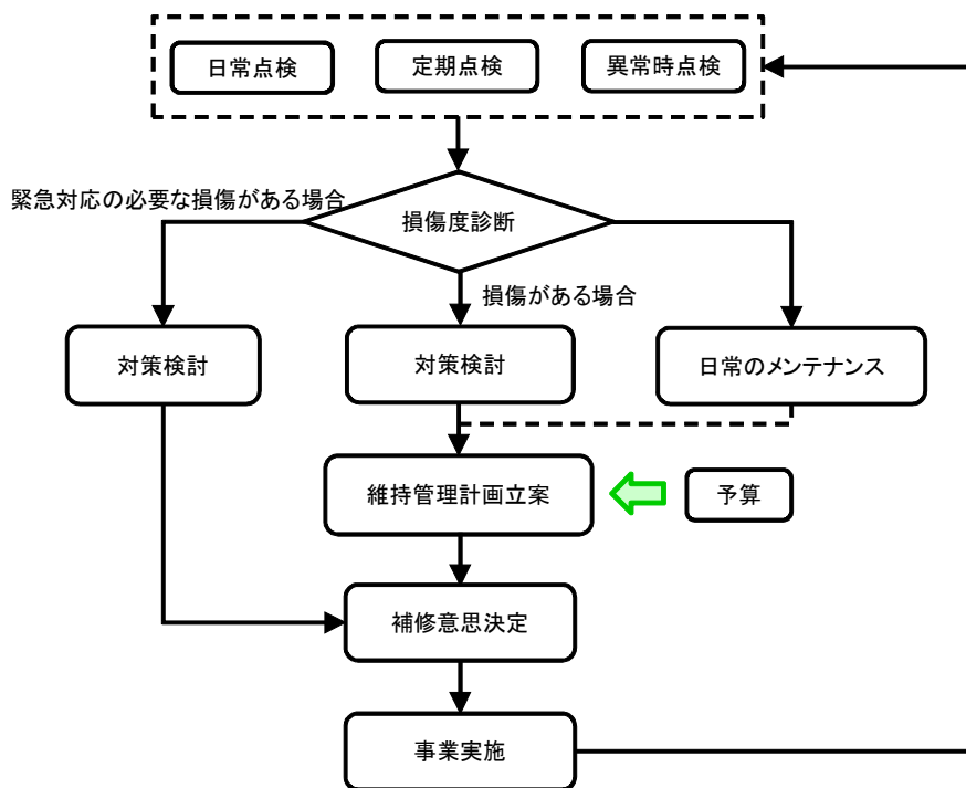
図. 5-1 橋梁維持管理の体系
