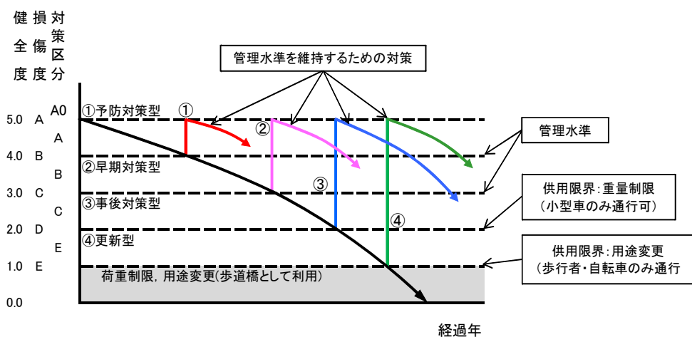
図. 7-1 シナリオごとの対策時期の設定
